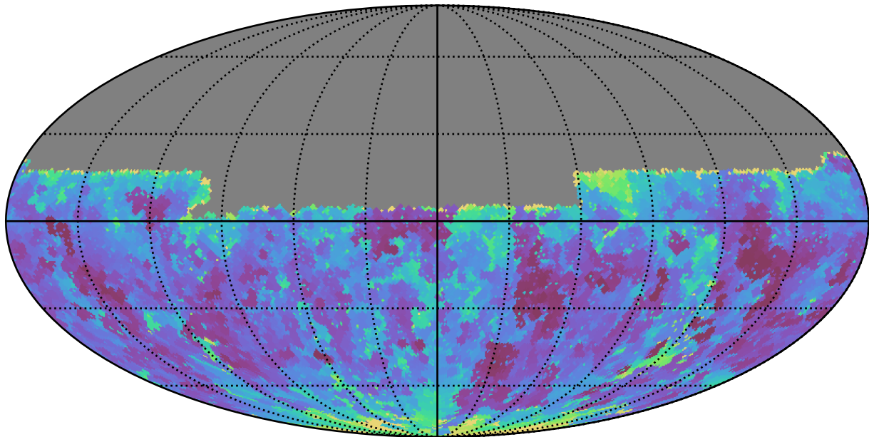
weather_cloudso18v3.4_10yrs Yr 1 y band: Min seeingGeom
