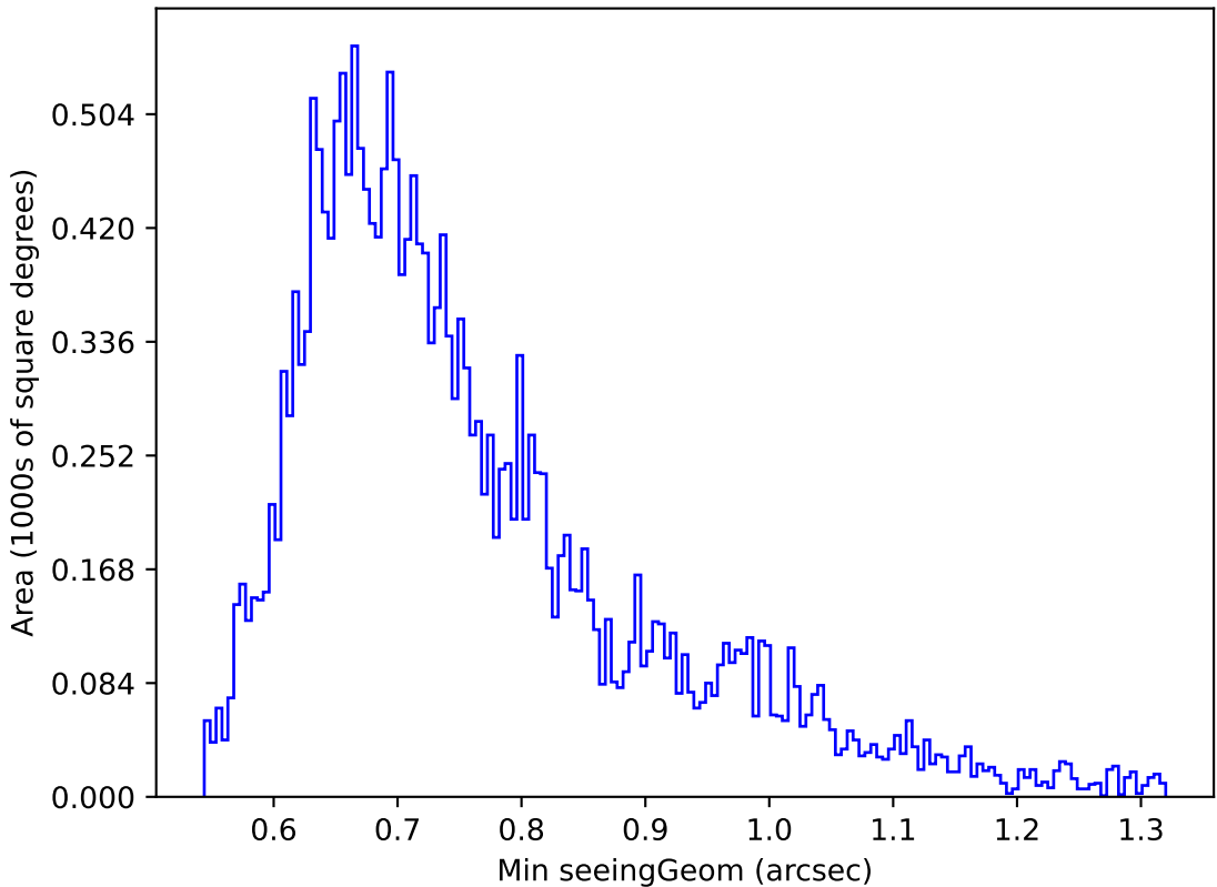
weather_cloudso18v3.4_10yrs Yr 1 u band: Min seeingGeom
