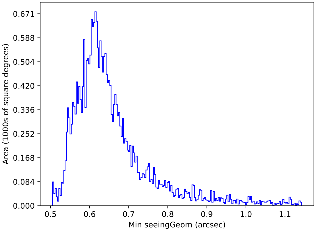
weather_cloudso18v3.4_10yrs Yr 1 r band: Min seeingGeom
