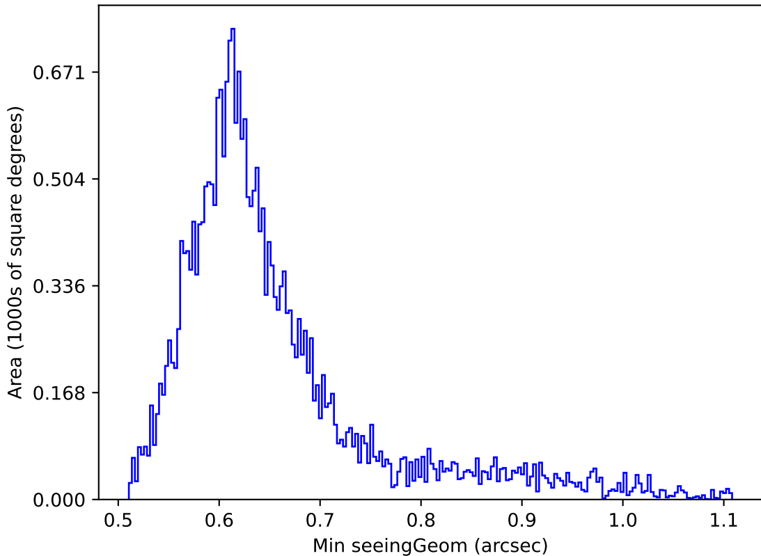
weather_cloudso18v3.4_10yrs Yr 1 i band: Min seeingGeom
