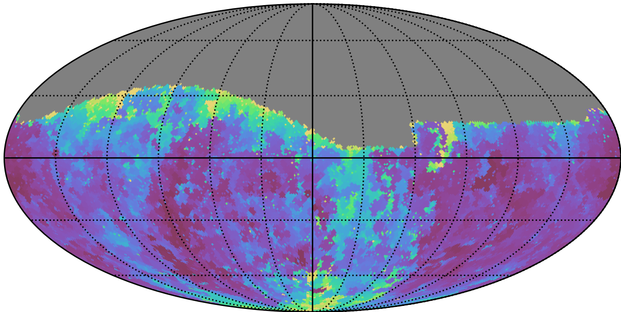
weather_cloudso18v3.4_10yrs Yr 1 g band: Min seeingGeom
