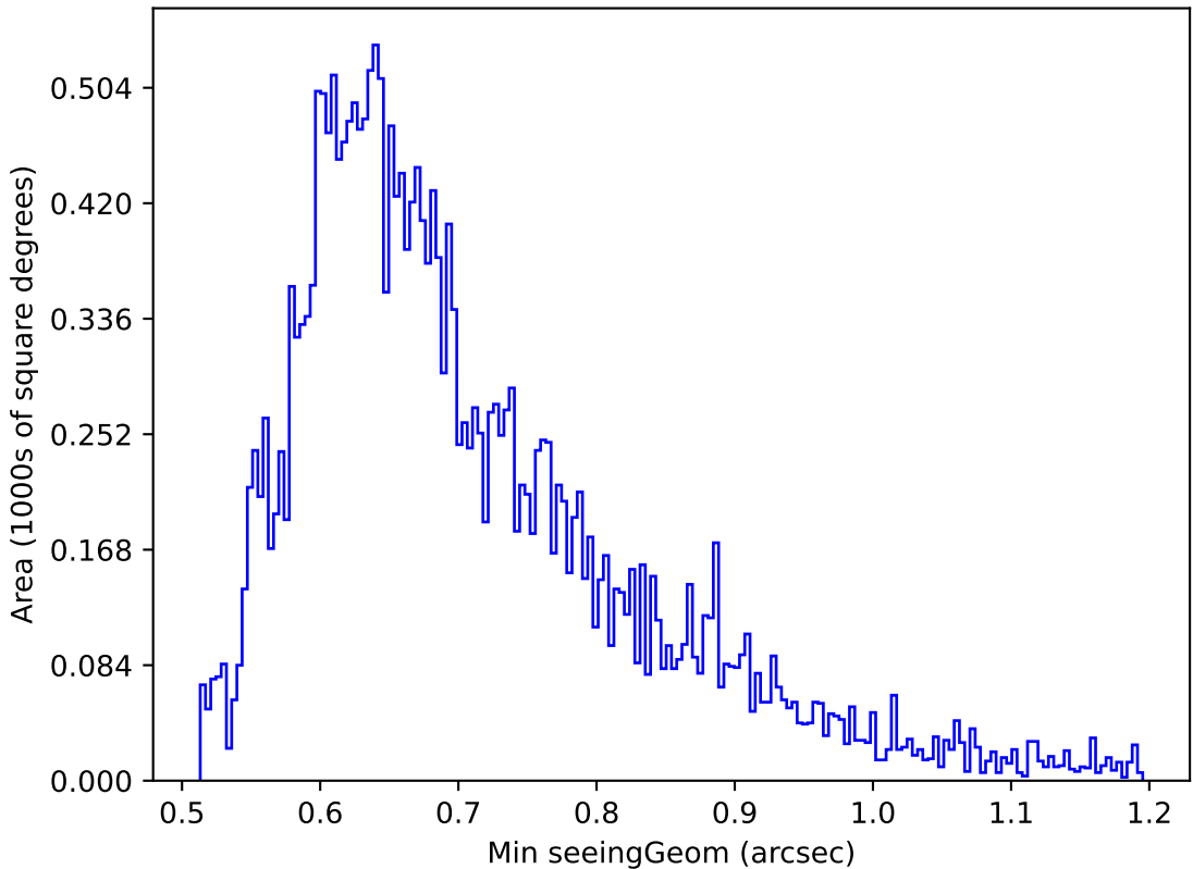
weather_cloudso18v3.4_10yrs Yr 1 g band: Min seeingGeom
