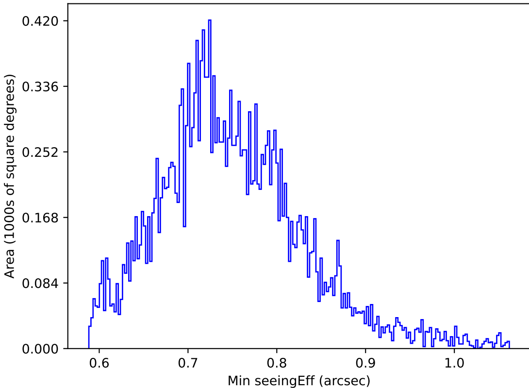
weather_cloudso18v3.4_10yrs Yr 1 y band: Min seeingEff
