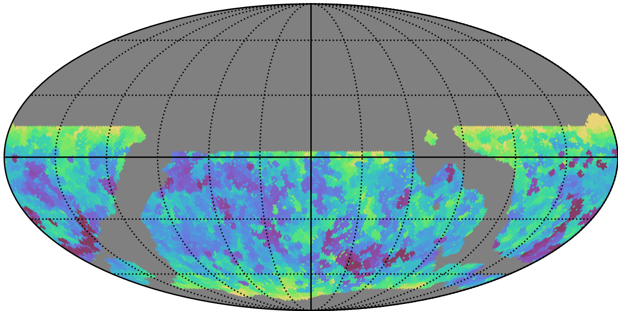
weather_cloudso18v3.4_10yrs WFD z band: Min seeingEff
