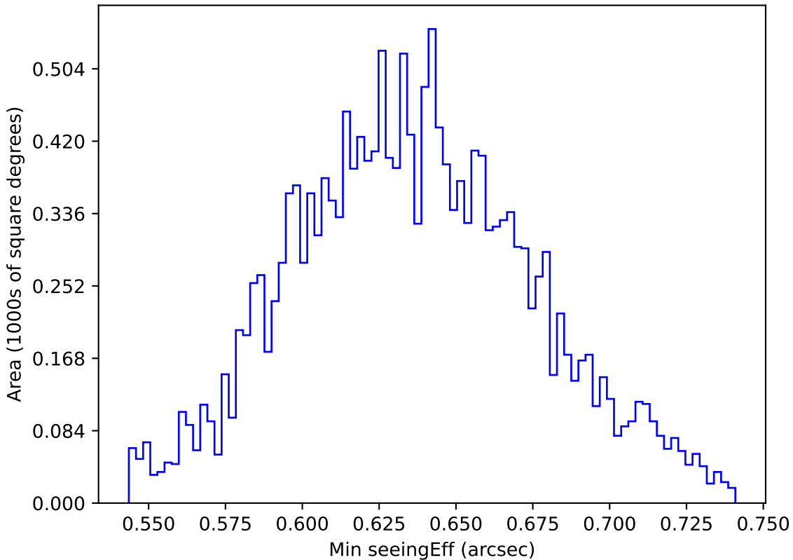
weather_cloudso18v3.4_10yrs WFD y band: Min seeingEff
