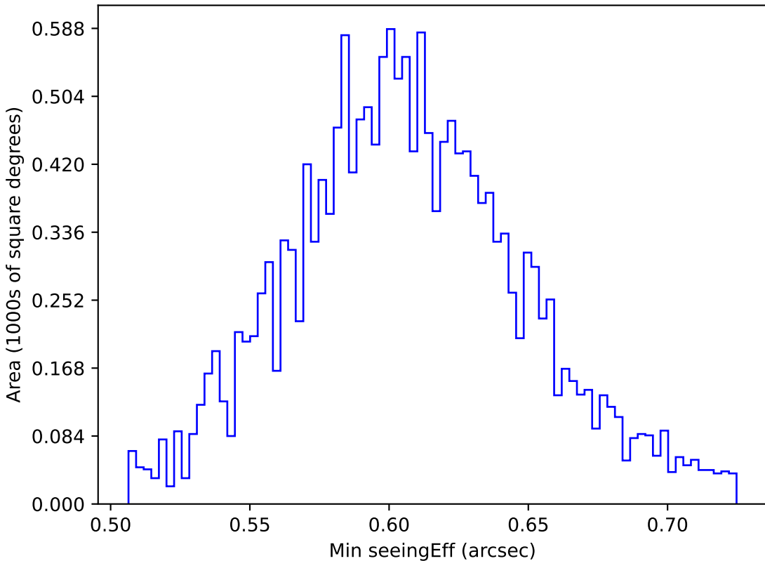
weather_cloudso18v3.4_10yrs WFD i band: Min seeingEff
