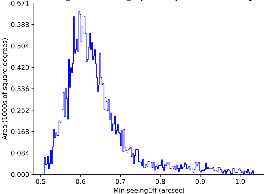
weather_cloudso18v3.4_10yrs All sky i band: Min seeingEff
