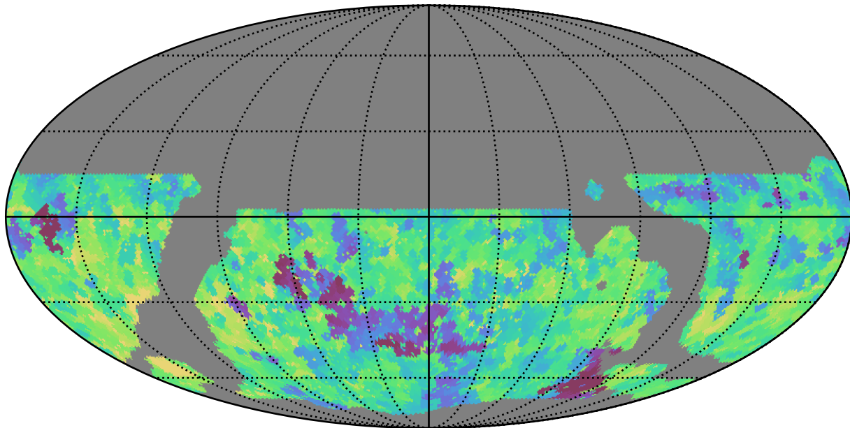
weather_cloudso18v3.4_10yrs WFD z band: Min saturation_mag
