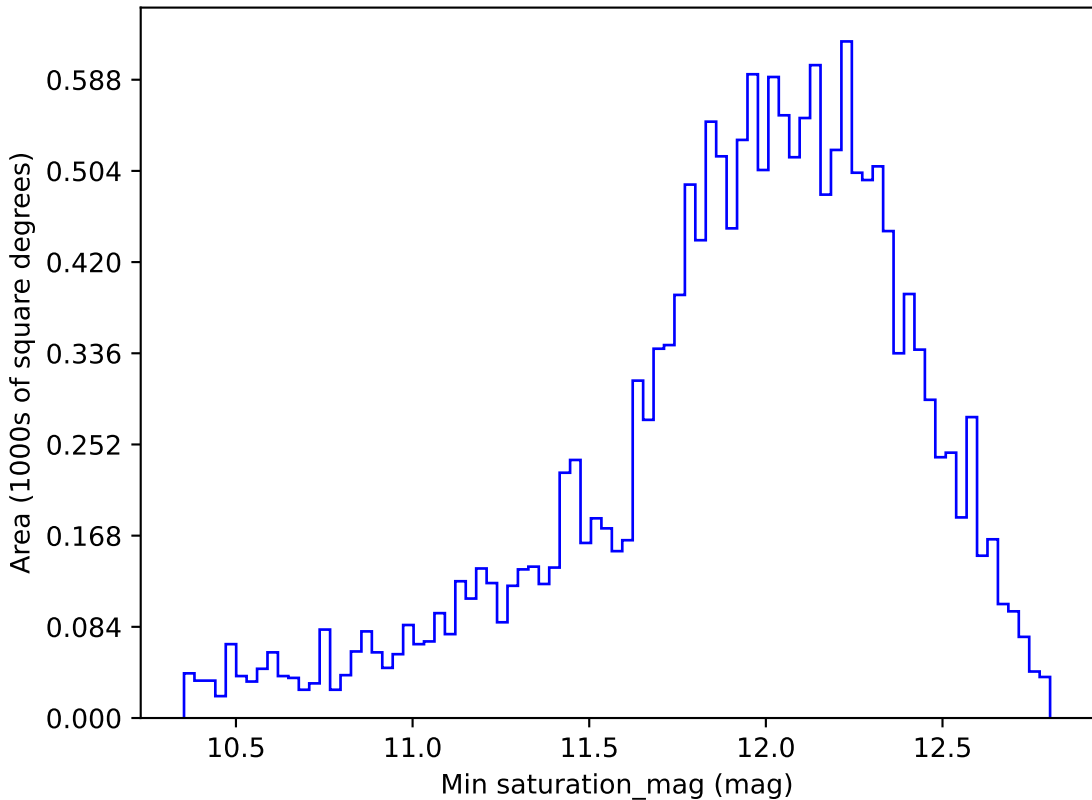
weather_cloudso18v3.4_10yrs WFD z band: Min saturation_mag
