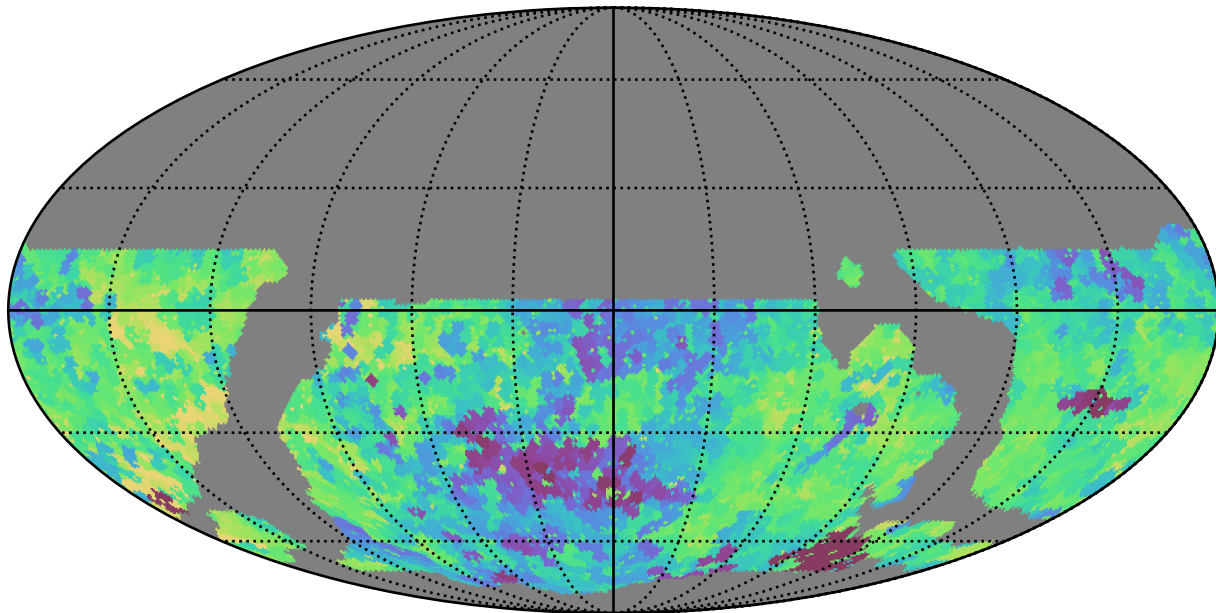
weather_cloudso18v3.4_10yrs WFD y band: Min saturation_mag
