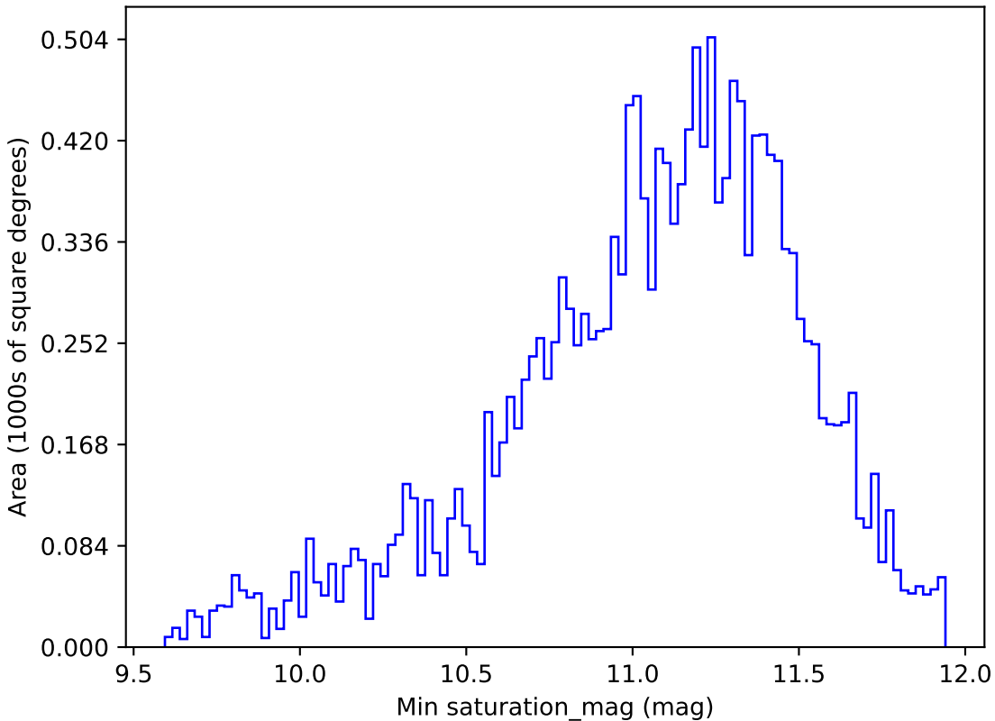
weather_cloudso18v3.4_10yrs WFD y band: Min saturation_mag
