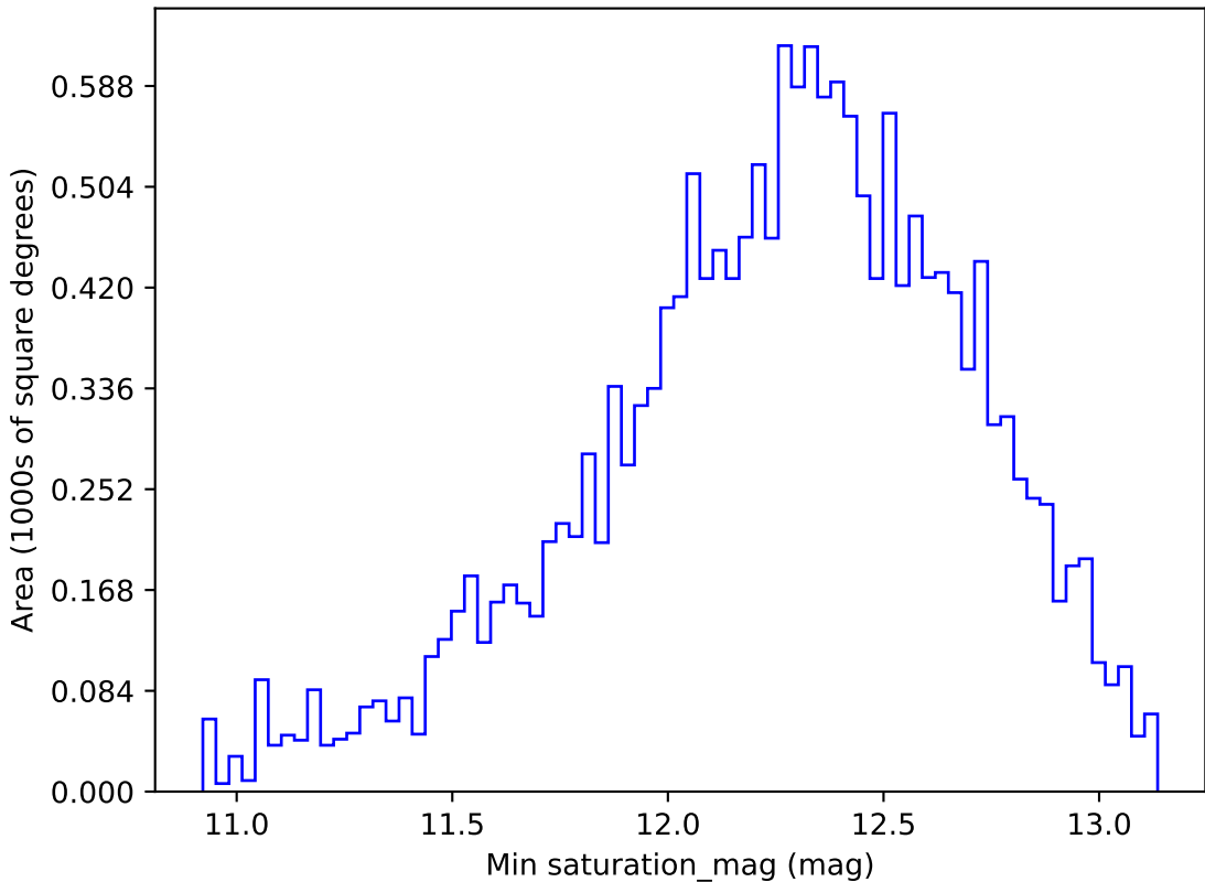
weather_cloudso18v3.4_10yrs WFD i band: Min saturation_mag
