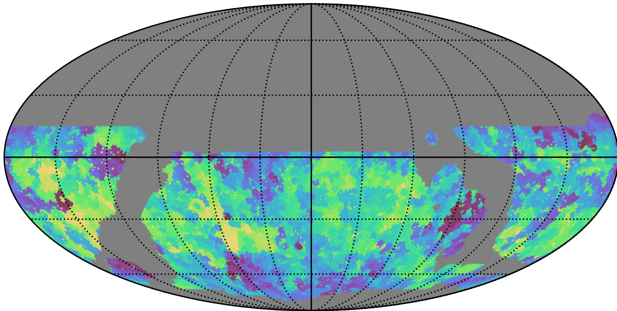
weather_cloudso18v3.4_10yrs WFD g band: Min saturation_mag
