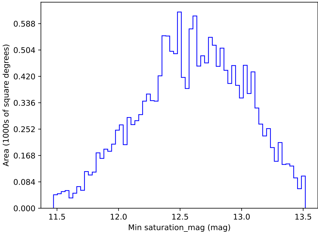
weather_cloudso18v3.4_10yrs WFD g band: Min saturation_mag
