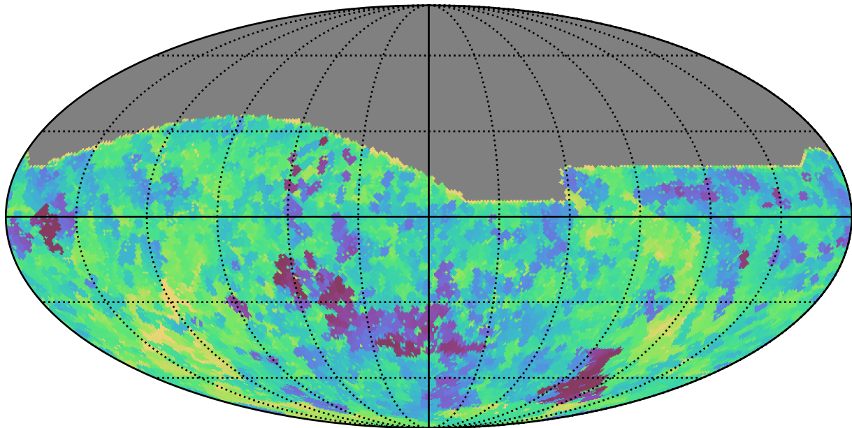
weather_cloudso18v3.4_10yrs All sky z band: Min saturation_mag
