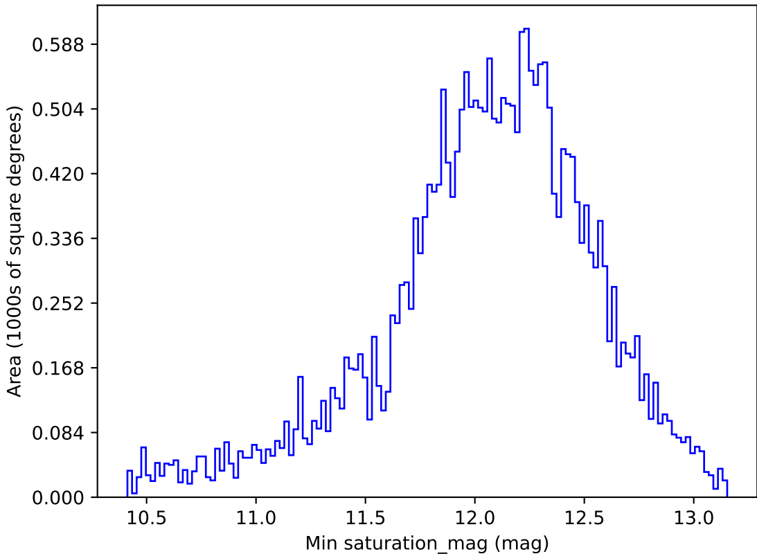
weather_cloudso18v3.4_10yrs All sky z band: Min saturation_mag
