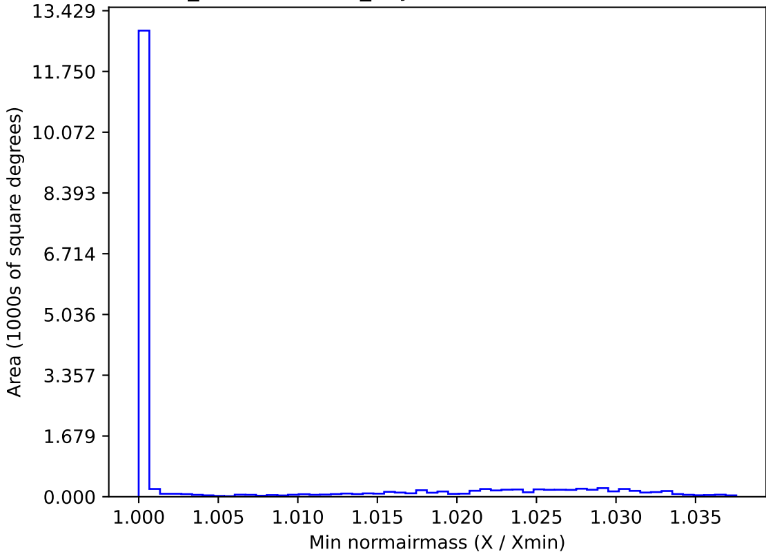
weather_cloudso18v3.4_10yrs WFD z band: Min normairmass
