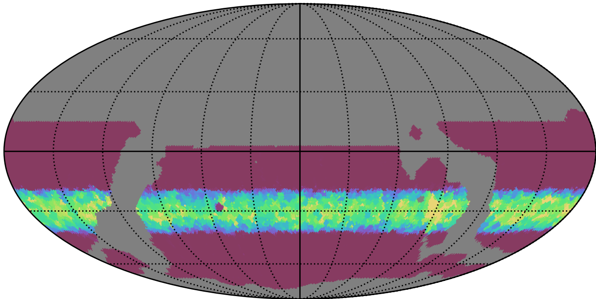
weather_cloudso18v3.4_10yrs WFD y band: Min normairmass
