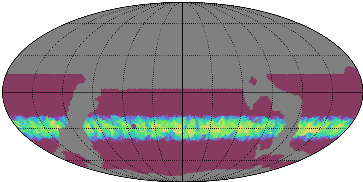
weather_cloudso18v3.4_10yrs WFD r band: Min normairmass
