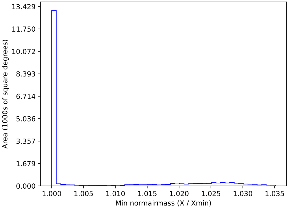
weather_cloudso18v3.4_10yrs WFD i band: Min normairmass
