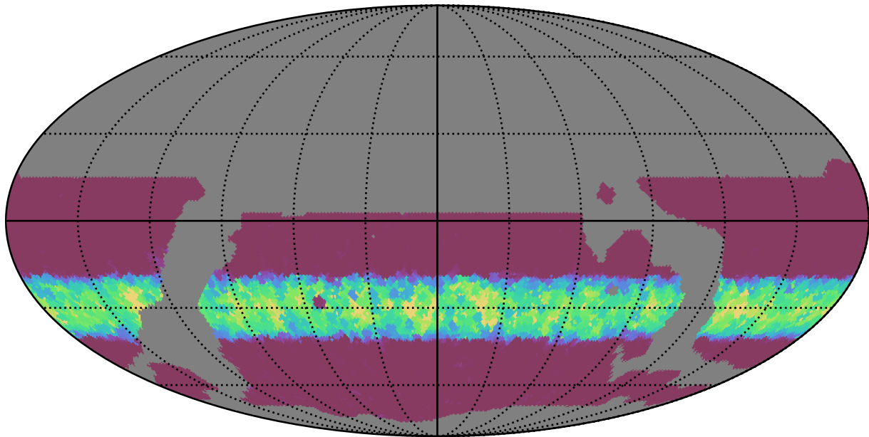
weather_cloudso18v3.4_10yrs WFD g band: Min normairmass
