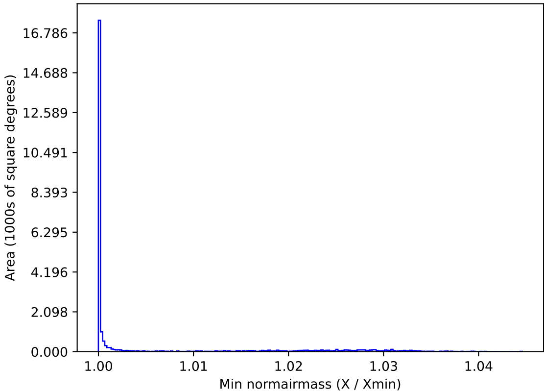
weather_cloudso18v3.4_10yrs All sky z band: Min normairmass
