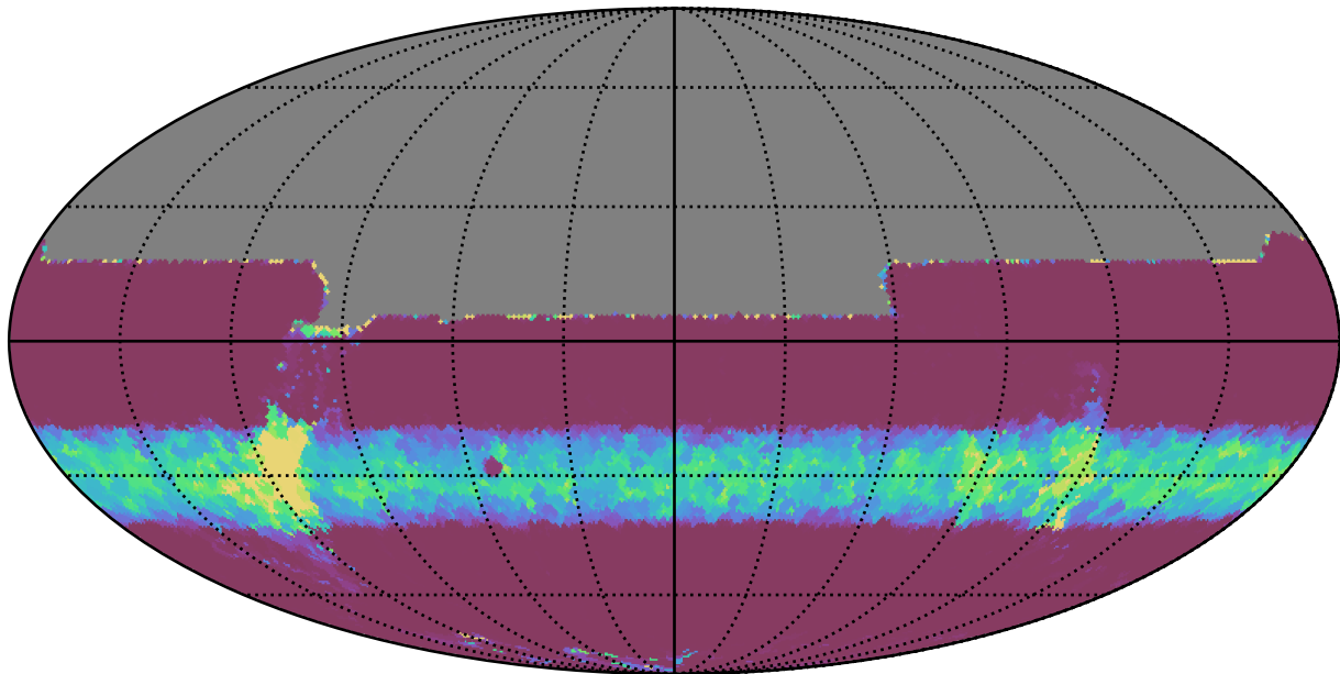
weather_cloudso18v3.4_10yrs All sky y band: Min normairmass
