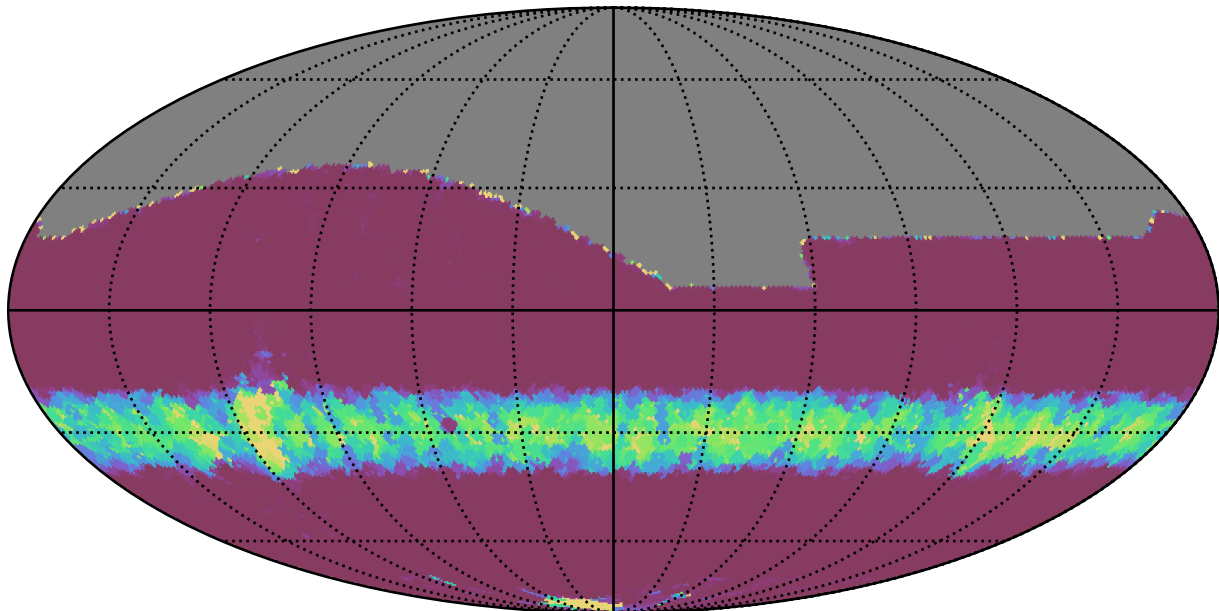
weather_cloudso18v3.4_10yrs All sky r band: Min normairmass
