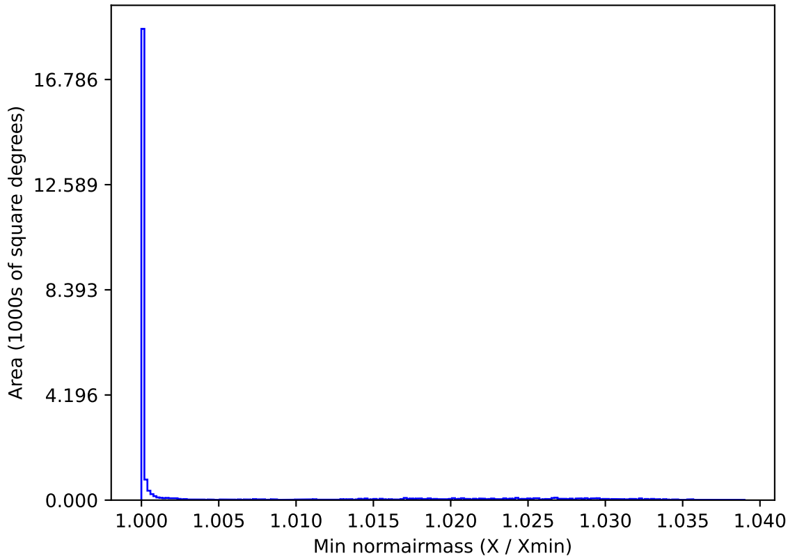
weather_cloudso18v3.4_10yrs All sky r band: Min normairmass
