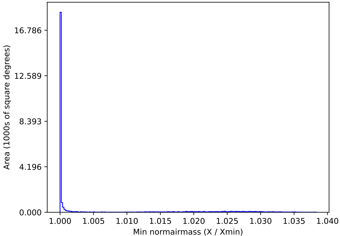
weather_cloudso18v3.4_10yrs All sky i band: Min normairmass
