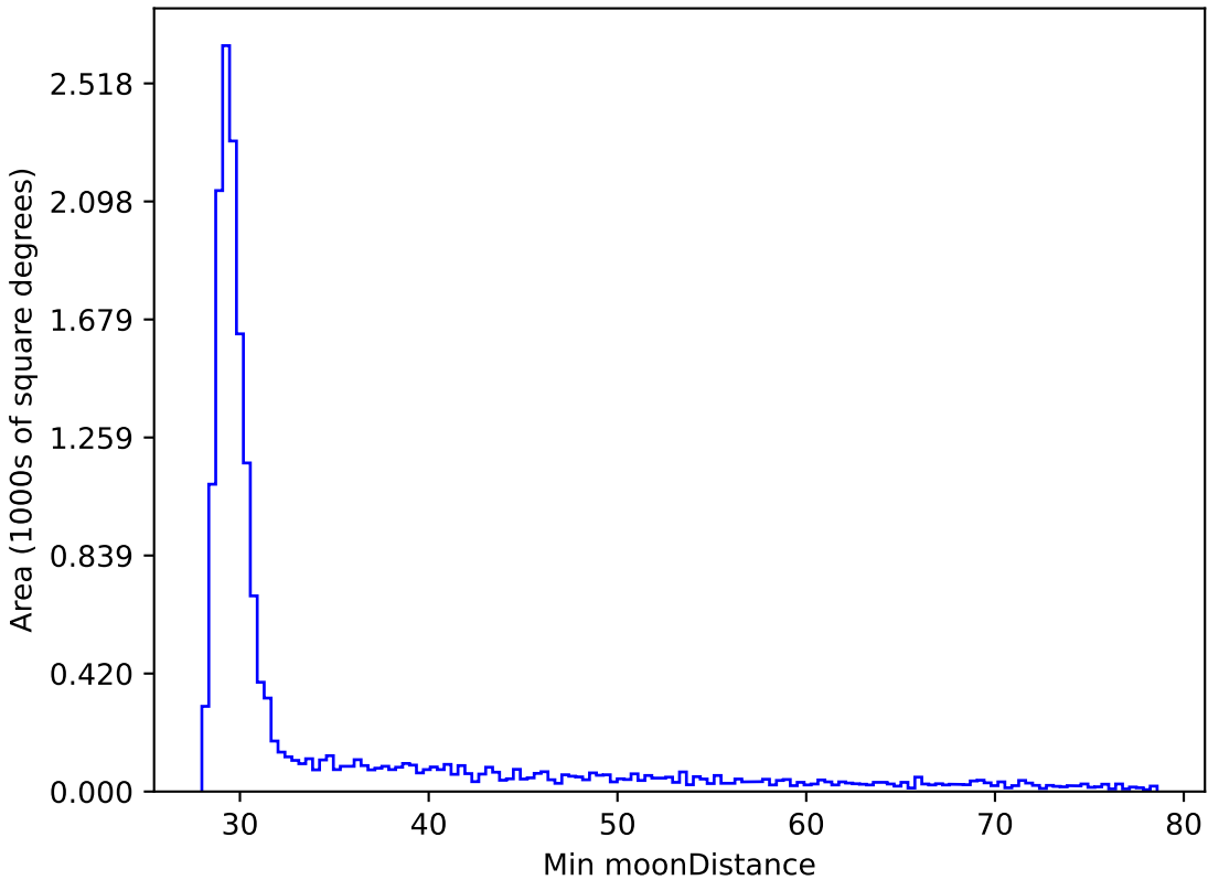
weather_cloudso18v3.4_10yrs WFD y band: Min moonDistance
