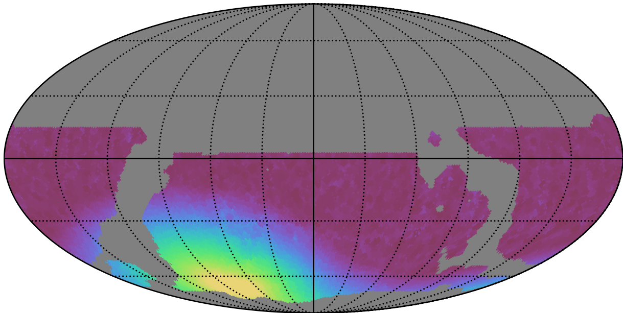
weather_cloudso18v3.4_10yrs WFD i band: Min moonDistance
