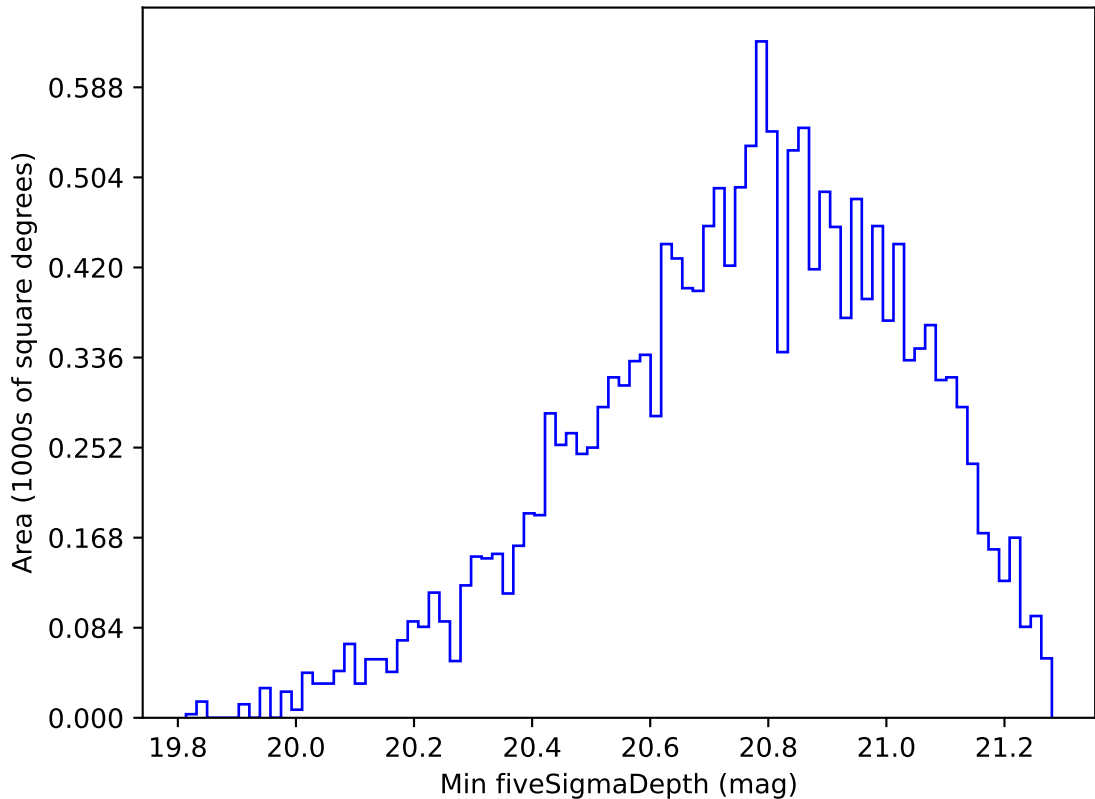
weather_cloudso18v3.4_10yrs WFD y band: Min fiveSigmaDepth
