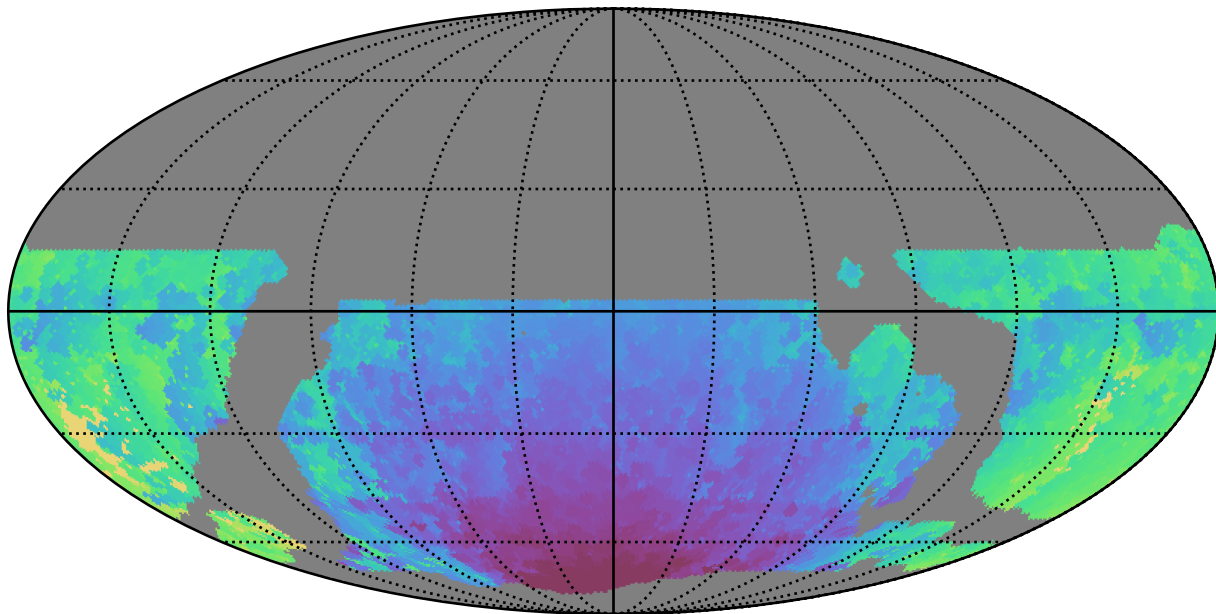
weather_cloudso18v3.4_10yrs WFD y band: Min HA
