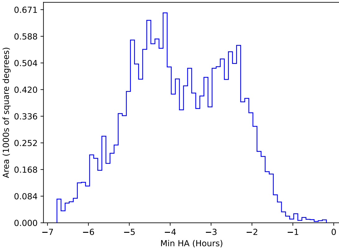
weather_cloudso18v3.4_10yrs WFD y band: Min HA
