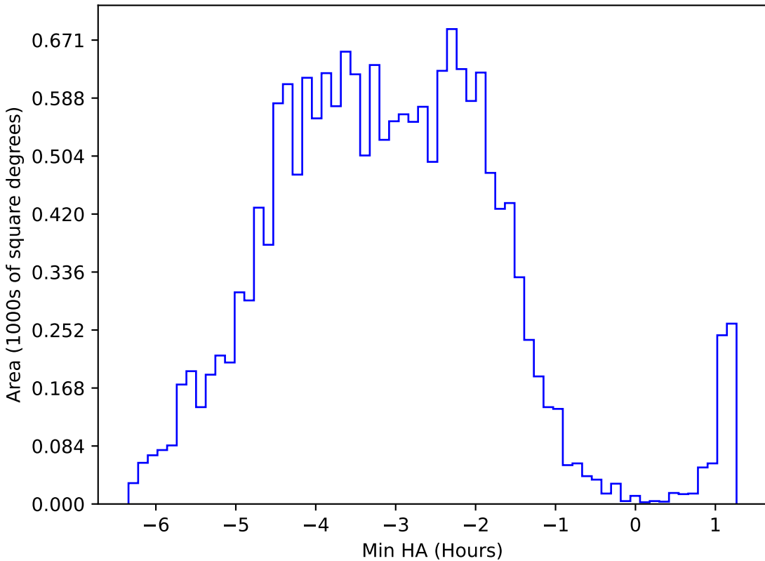
weather_cloudso18v3.4_10yrs WFD u band: Min HA
