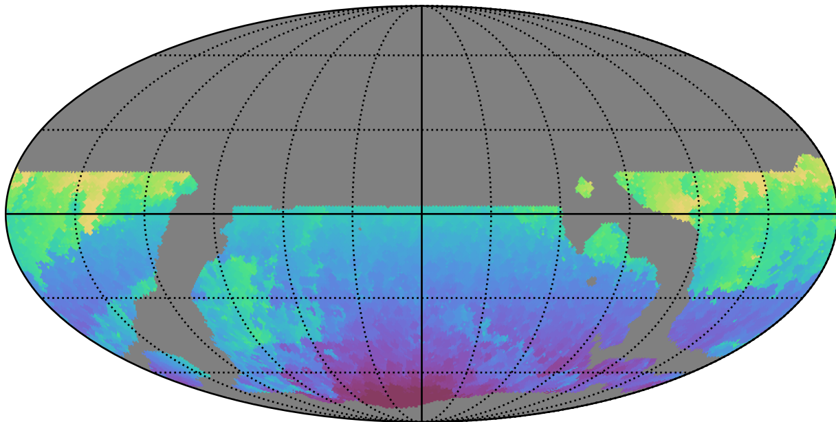
weather_cloudso18v3.4_10yrs WFD r band: Min HA
