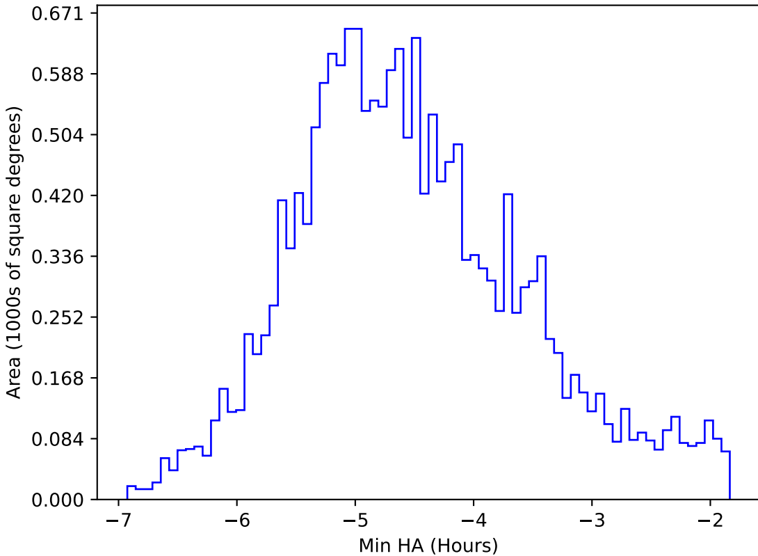
weather_cloudso18v3.4_10yrs WFD r band: Min HA
