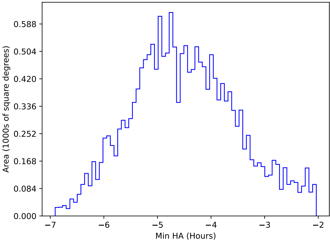
weather_cloudso18v3.4_10yrs WFD i band: Min HA
