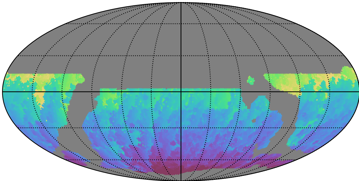
weather_cloudso18v3.4_10yrs WFD g band: Min HA
