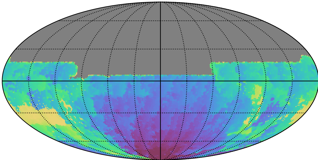
weather_cloudso18v3.4_10yrs All sky u band: Min HA
