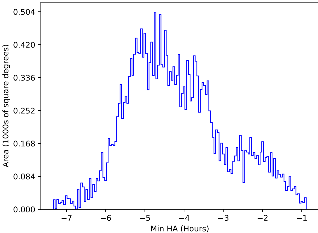
weather_cloudso18v3.4_10yrs All sky r band: Min HA
