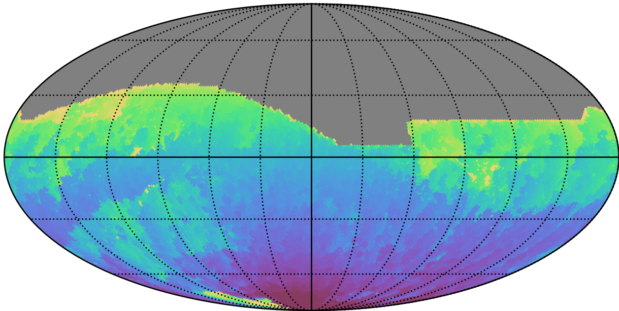
weather_cloudso18v3.4_10yrs All sky i band: Min HA
