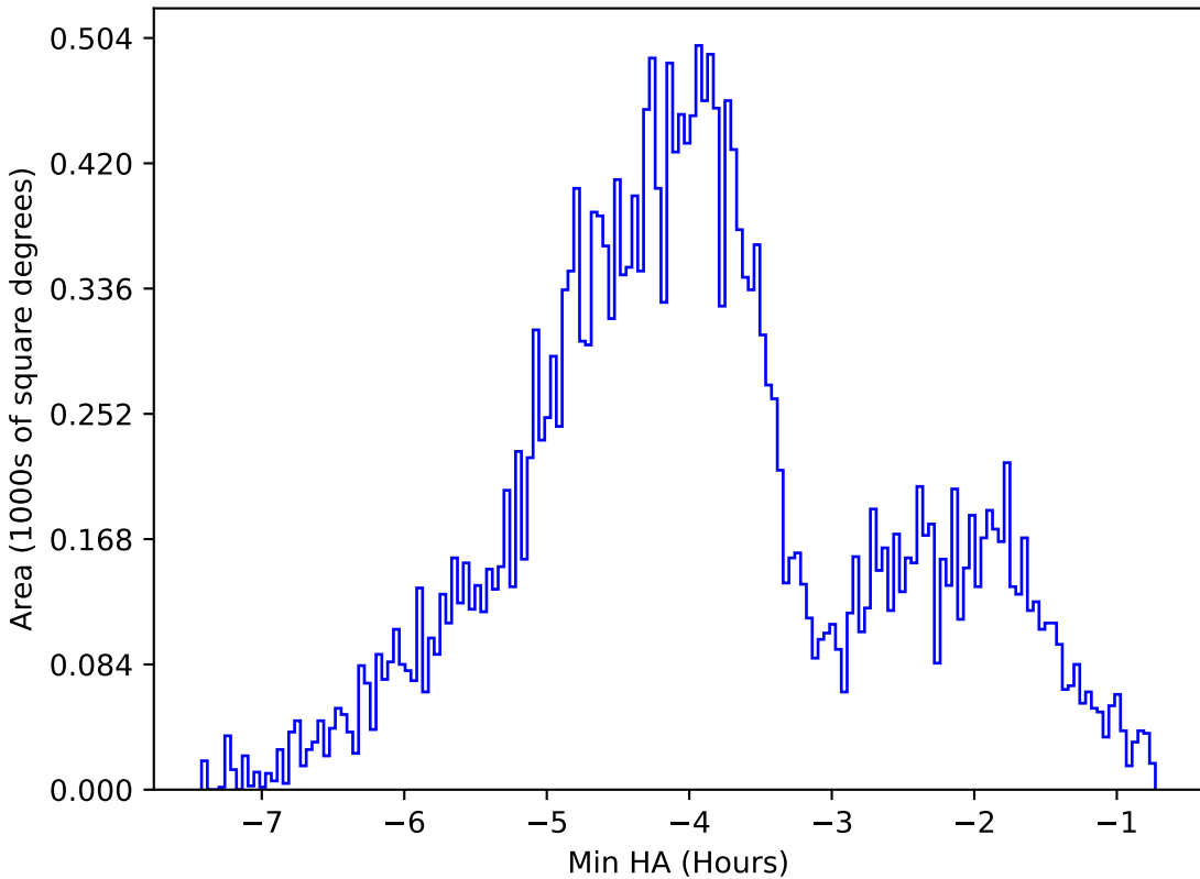
weather_cloudso18v3.4_10yrs All sky g band: Min HA
