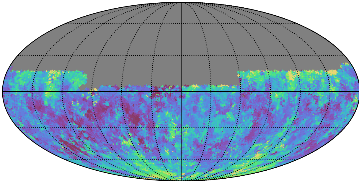
weather_cloudso18v3.4_10yrs Yr 1 y band: Median seeingGeom
