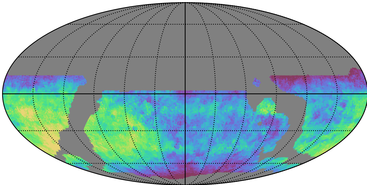
weather_cloudso18v3.4_10yrs WFD z band: Median saturation_mag
