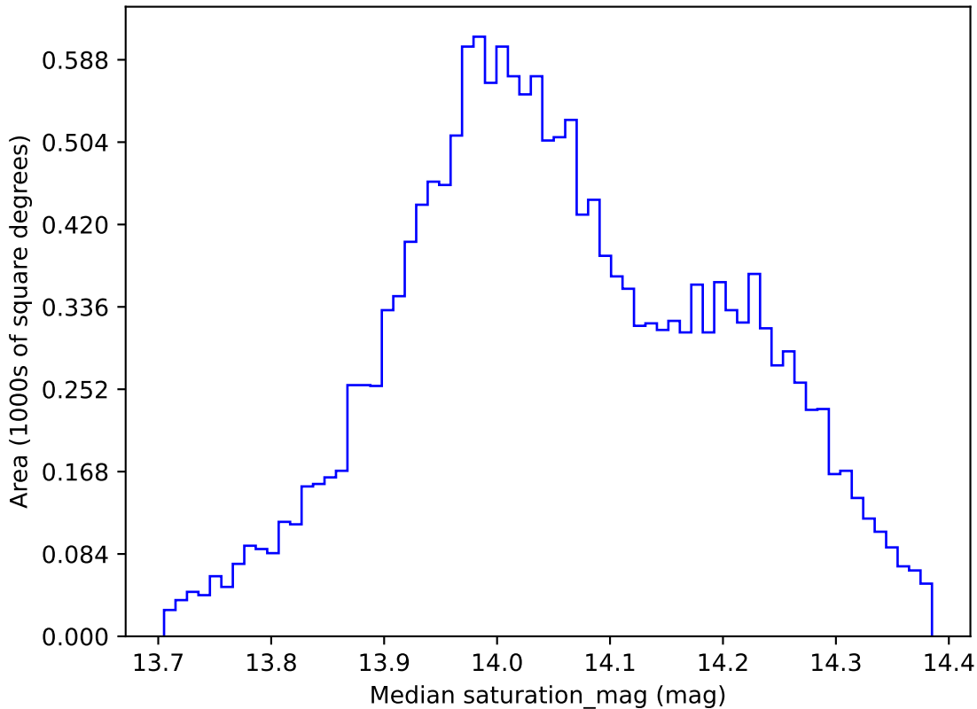
weather_cloudso18v3.4_10yrs WFD z band: Median saturation_mag
