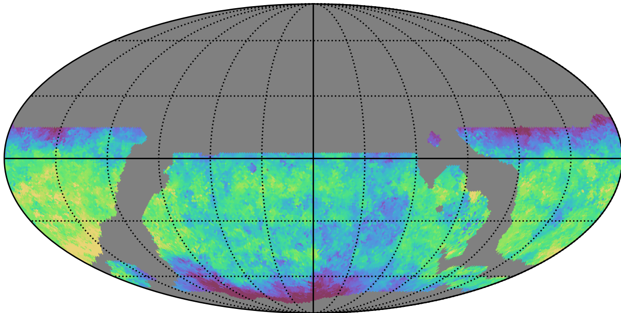
weather_cloudso18v3.4_10yrs WFD u band: Median saturation_mag
