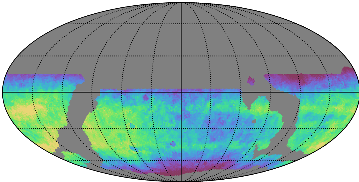
weather_cloudso18v3.4_10yrs WFD r band: Median saturation_mag
