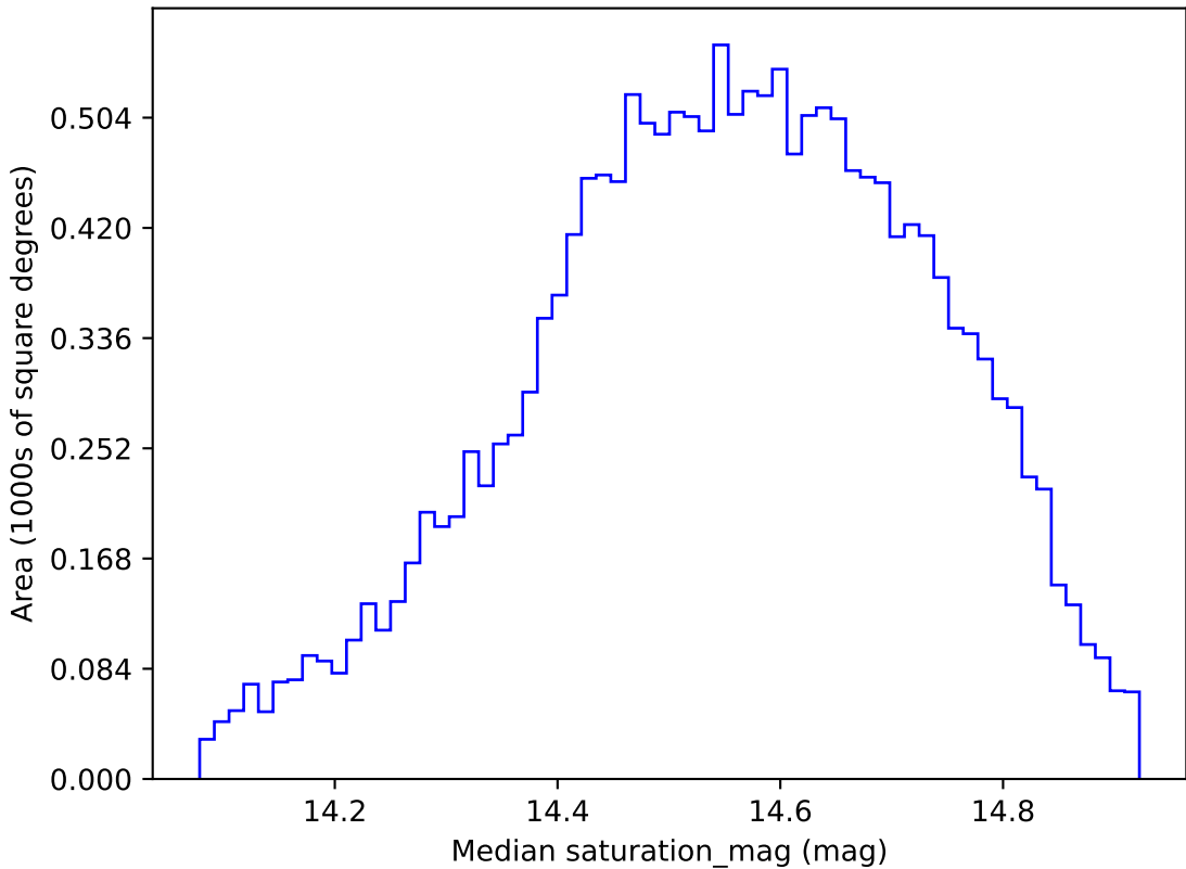
weather_cloudso18v3.4_10yrs WFD r band: Median saturation_mag
